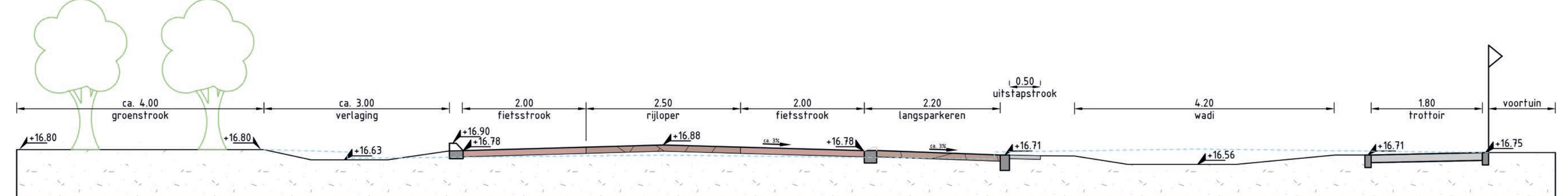
Doorsnede A-A
